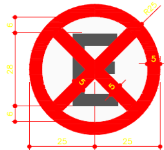
R-6c PROIBIDO PARAR E ESTACIONAR Fonte: Arial Narrow (Negrito) H da letra: 28,0cm
